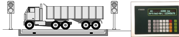
Einzel- oder Verbundwaage
