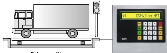
Fahrzeug-Waage
